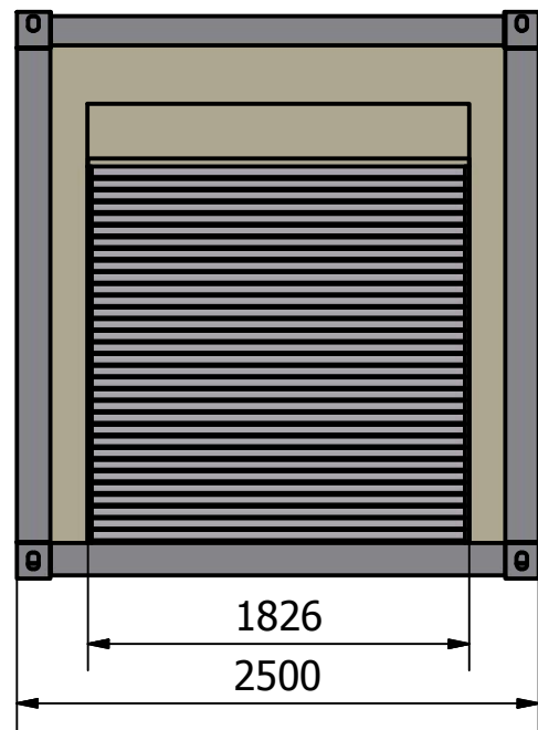
VISTA POSTERIOR ( 1 : 40 )
