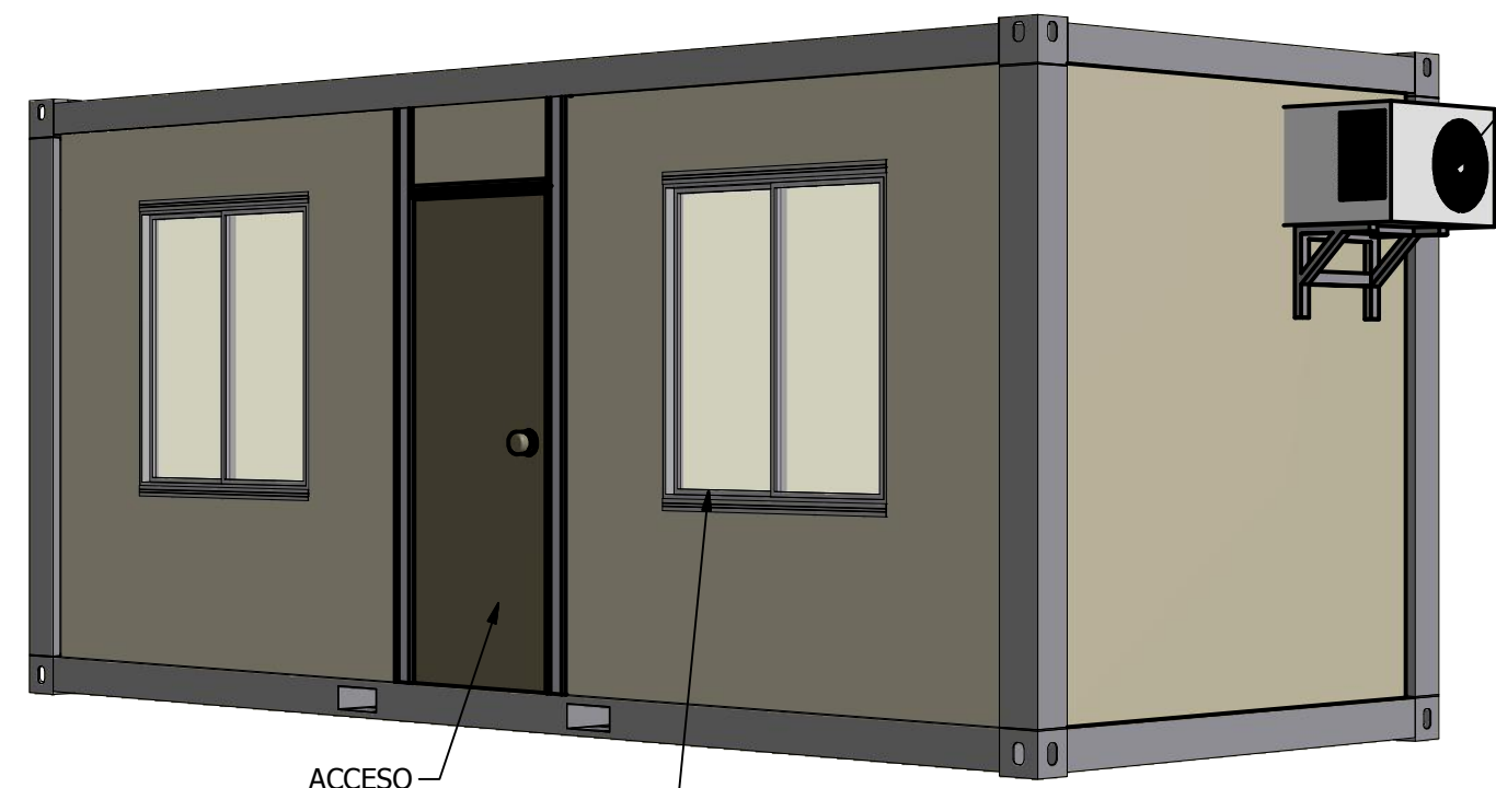
PERSPECTIVA ESCALA 1:35
