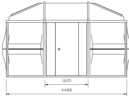
Elevación
