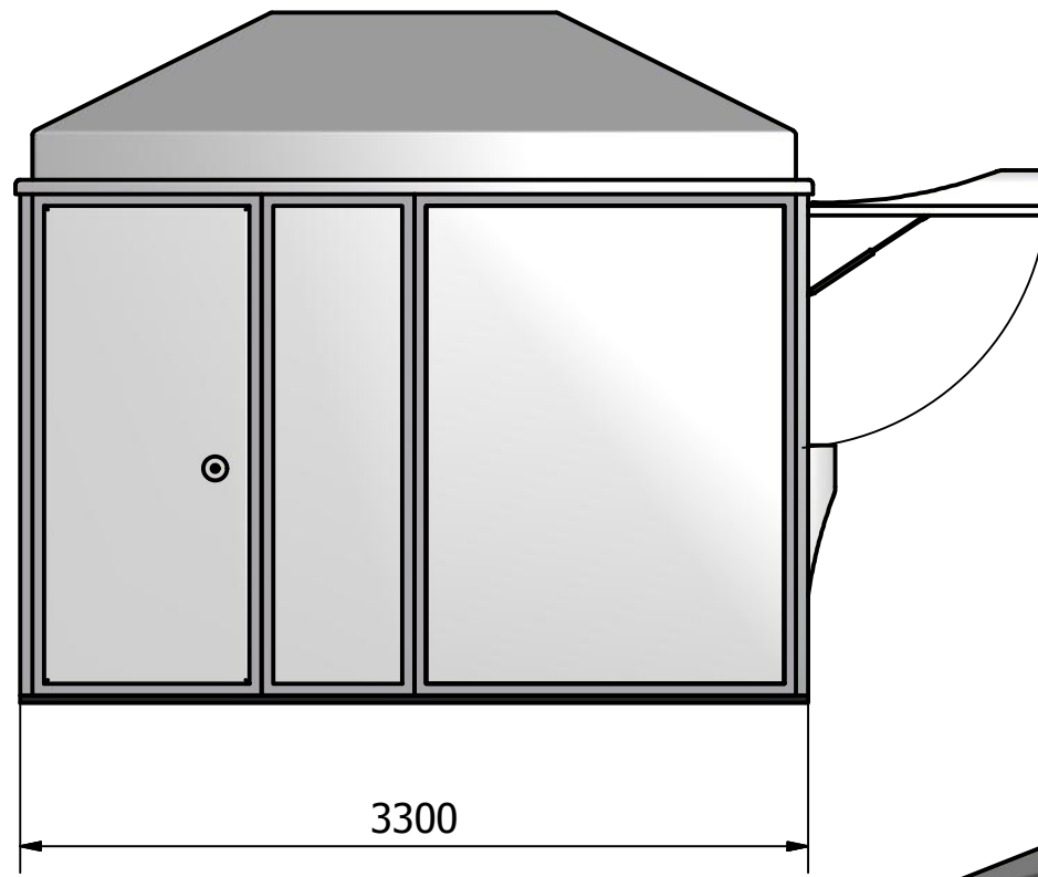
VISTA LATERAL IZQ. ( 1 : 35 )
